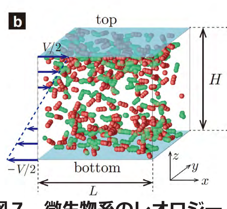
図7. 微生物系のレオロジー
