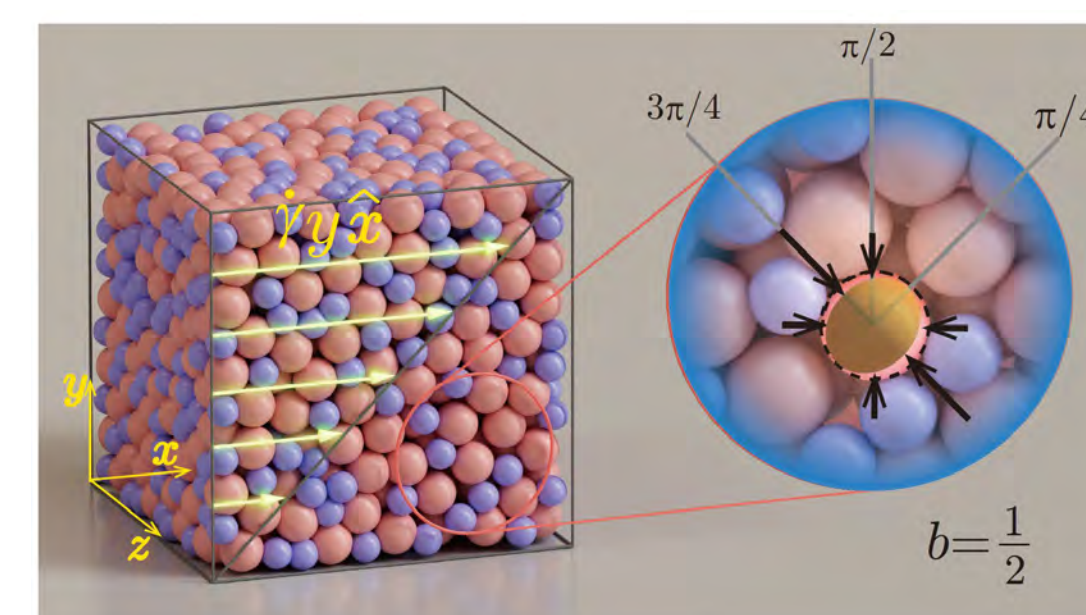
図4. 剪断流下における有効体積の概念図
