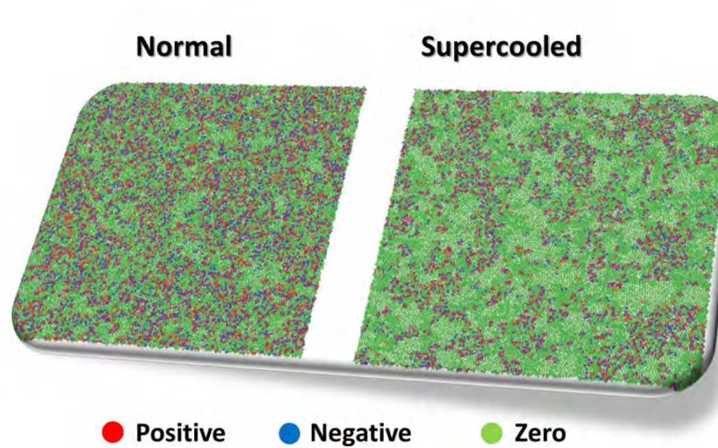
図1. 密度交換イベントの協同性 (左)ノーマルな液体(右)過冷却液体
