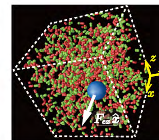
図9. (上)アクティブ流体におけるマイクロレオロジー (左)流体力学的相互作用による抵抗低減の概念図
