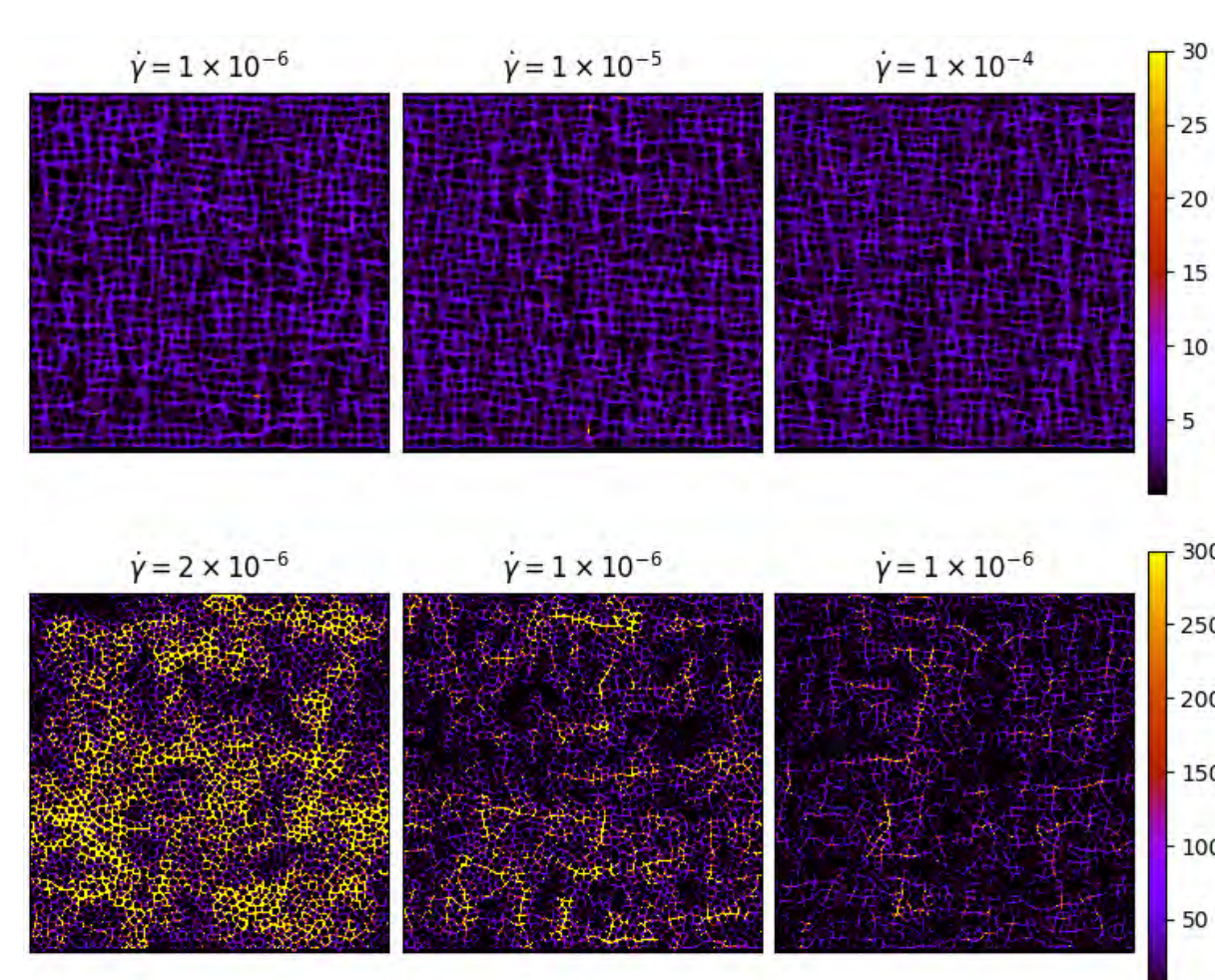
図3. 粉体懸濁液における溶媒散逸の空間相関
