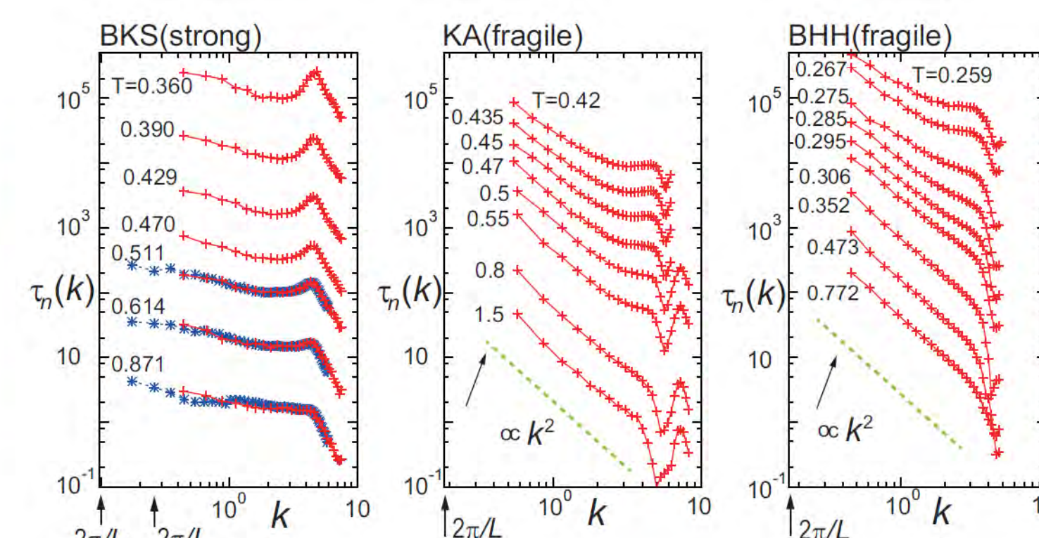
図2. 密度揺らぎの緩和時間の波数依存性
