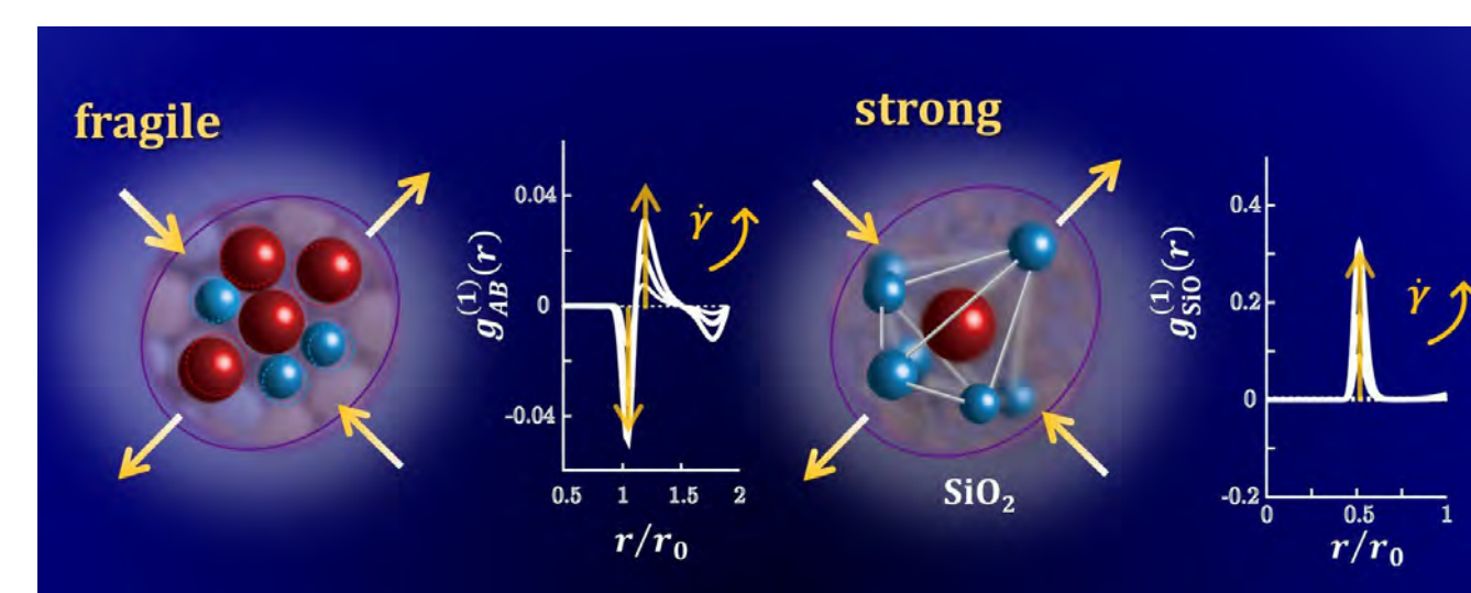
図5. 単純剪断流れ下の粒子配置
