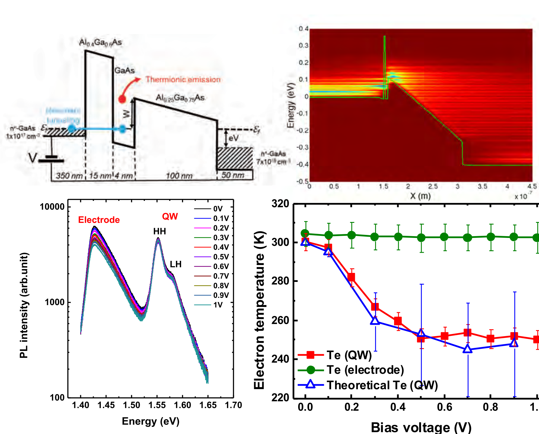
半導体ヘテロ構造を用いた熱電子冷却デバイス
