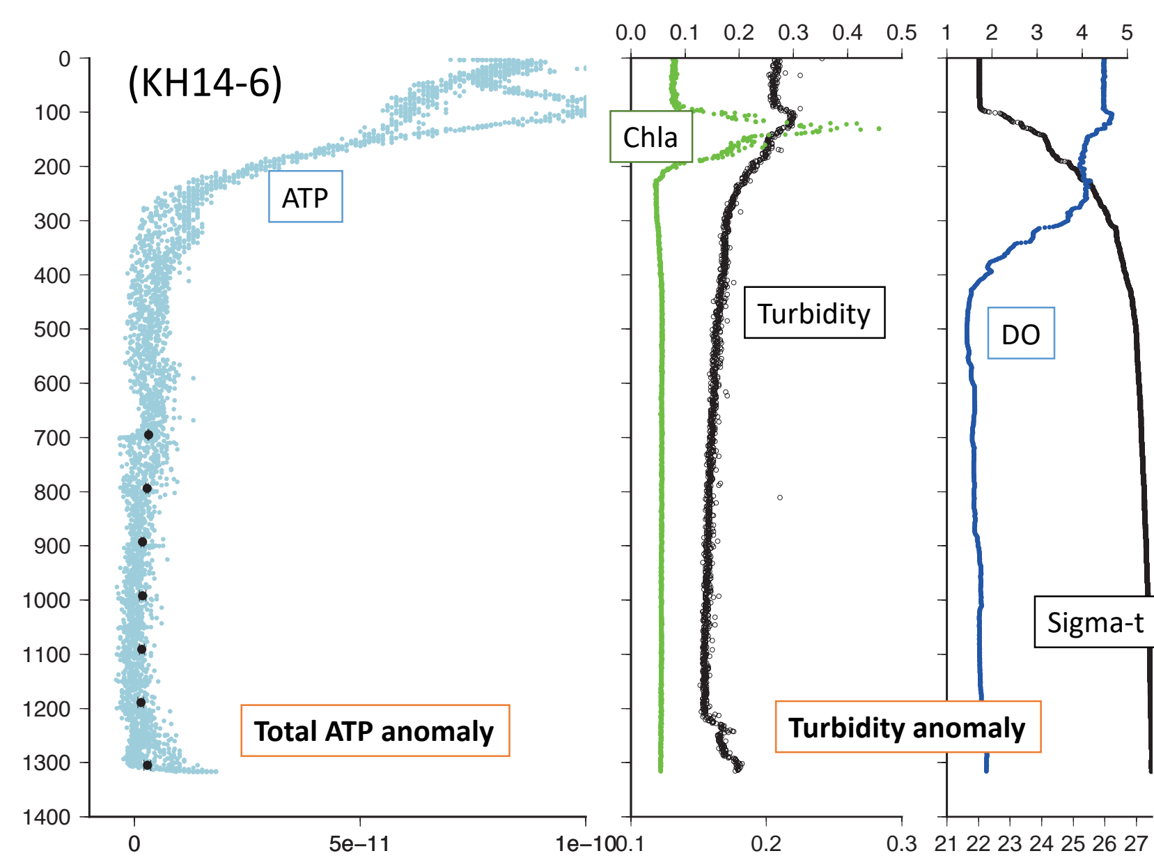
マリアナトラフ Seamont-Xにおける鉛直ATP計測の結果。ATP定量分析装置をCTDに搭載して計測
