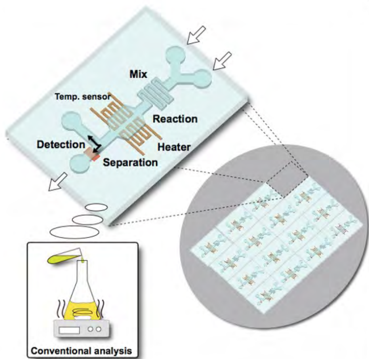
マイクロ流体システム概念図
