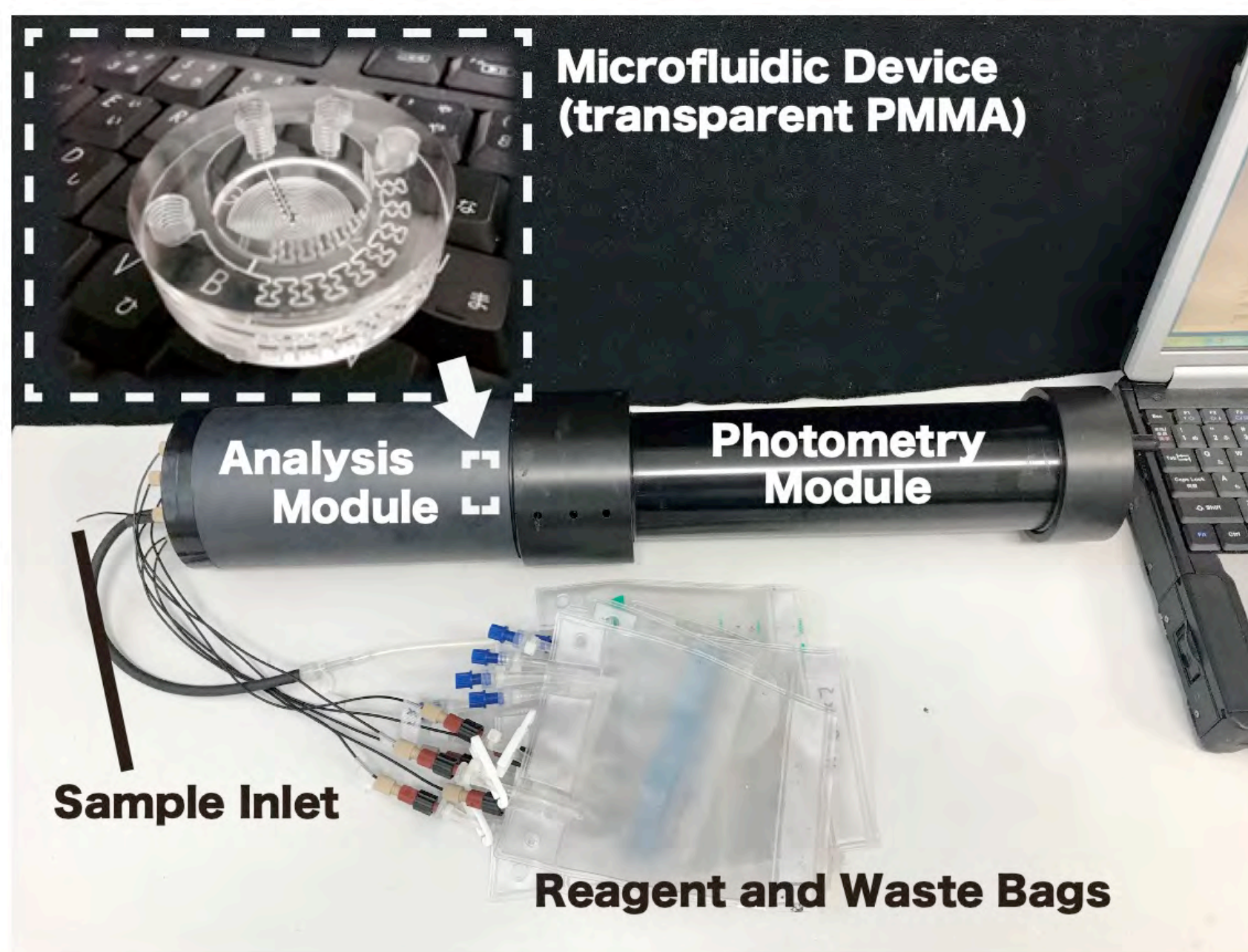
現場型 ATP定量分析装置の外観
