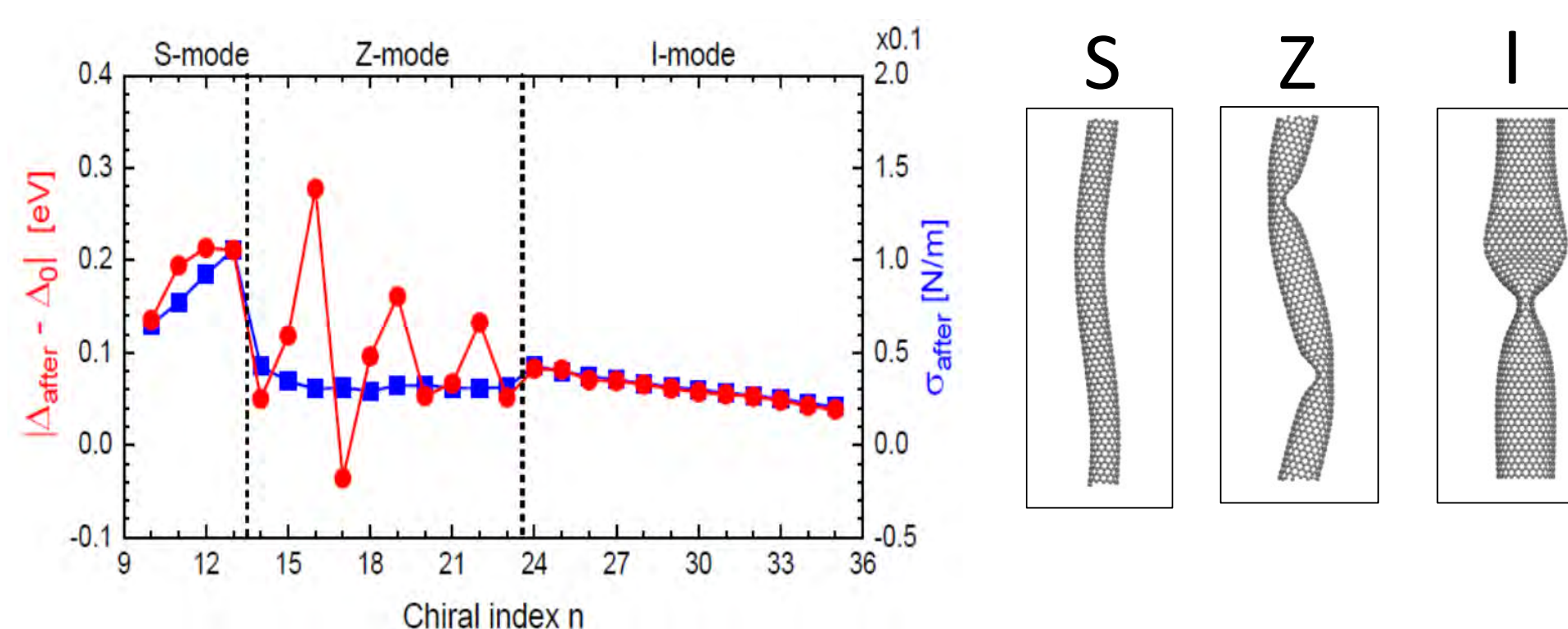
ナノチューブ径 (n) によって変化する座屈モード、および座屈によるバンドギャップ変化と座屈後荷重の相関性
