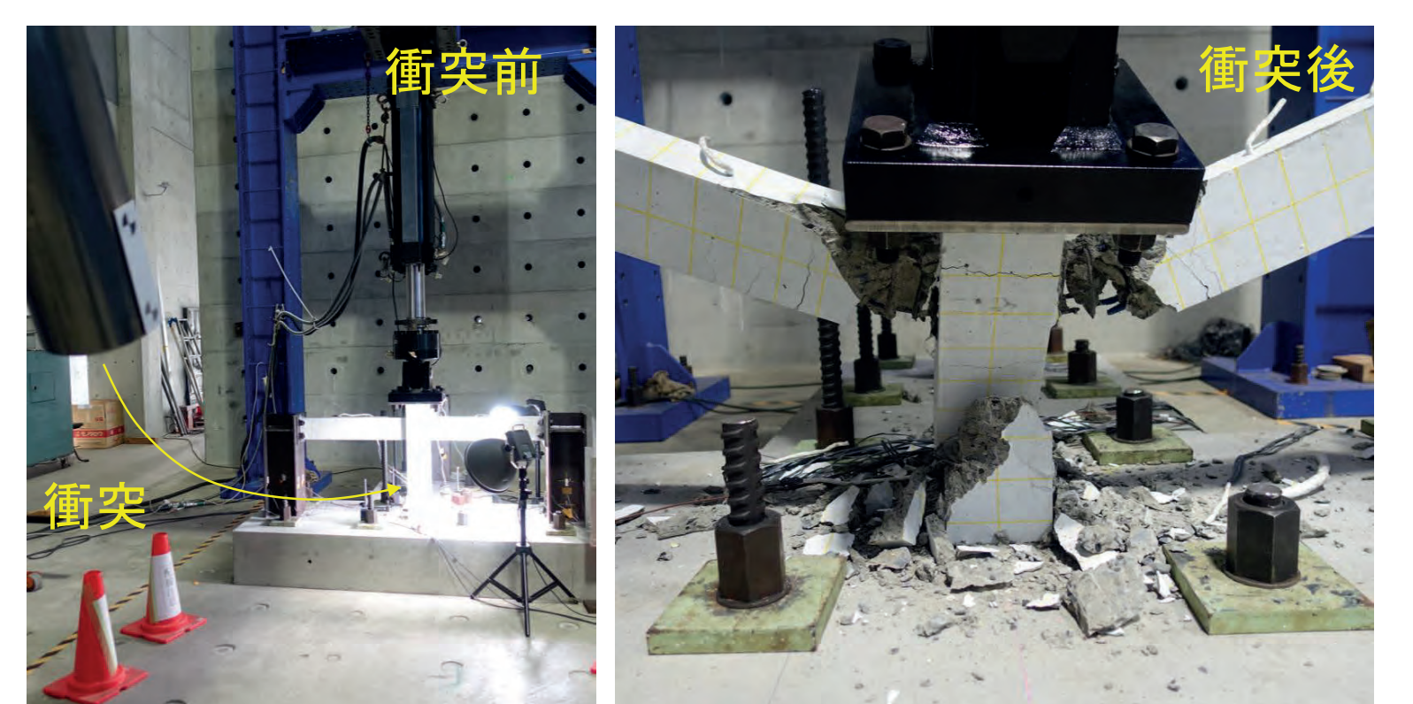
鉄筋コンクリート造架構への模擬船舶の衝突実験
