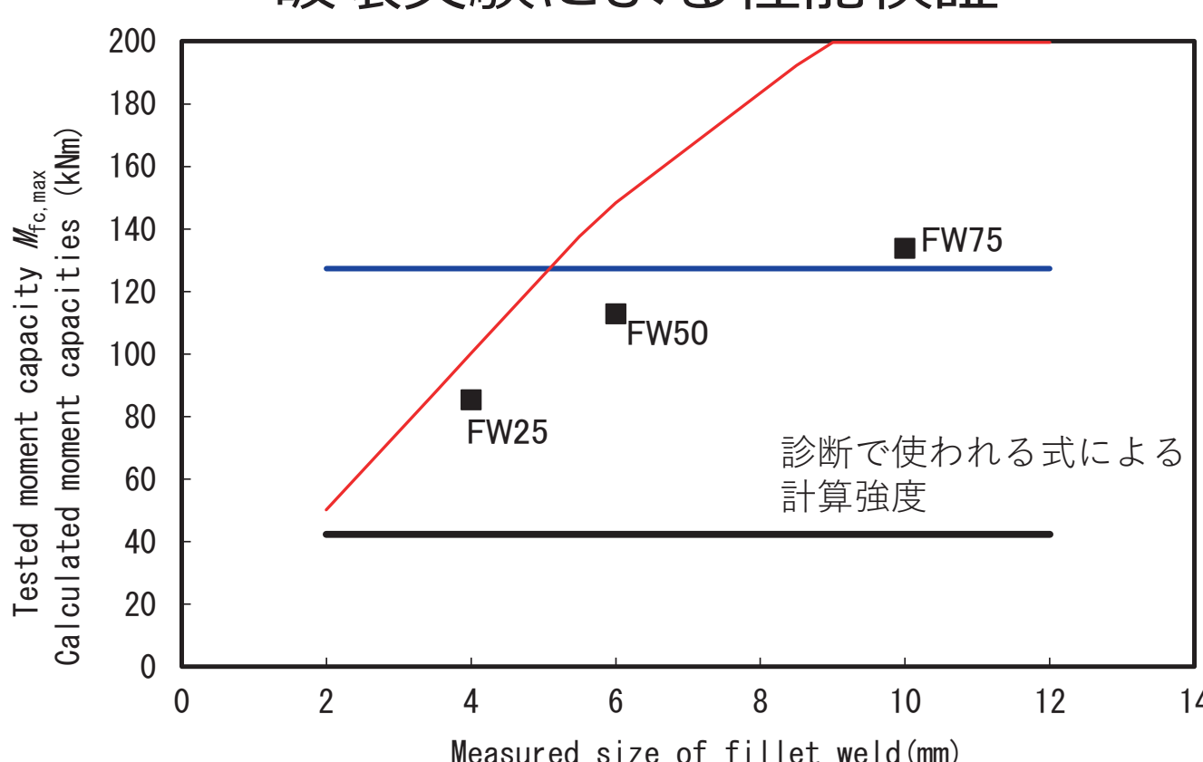
破壊実験による性能検証
