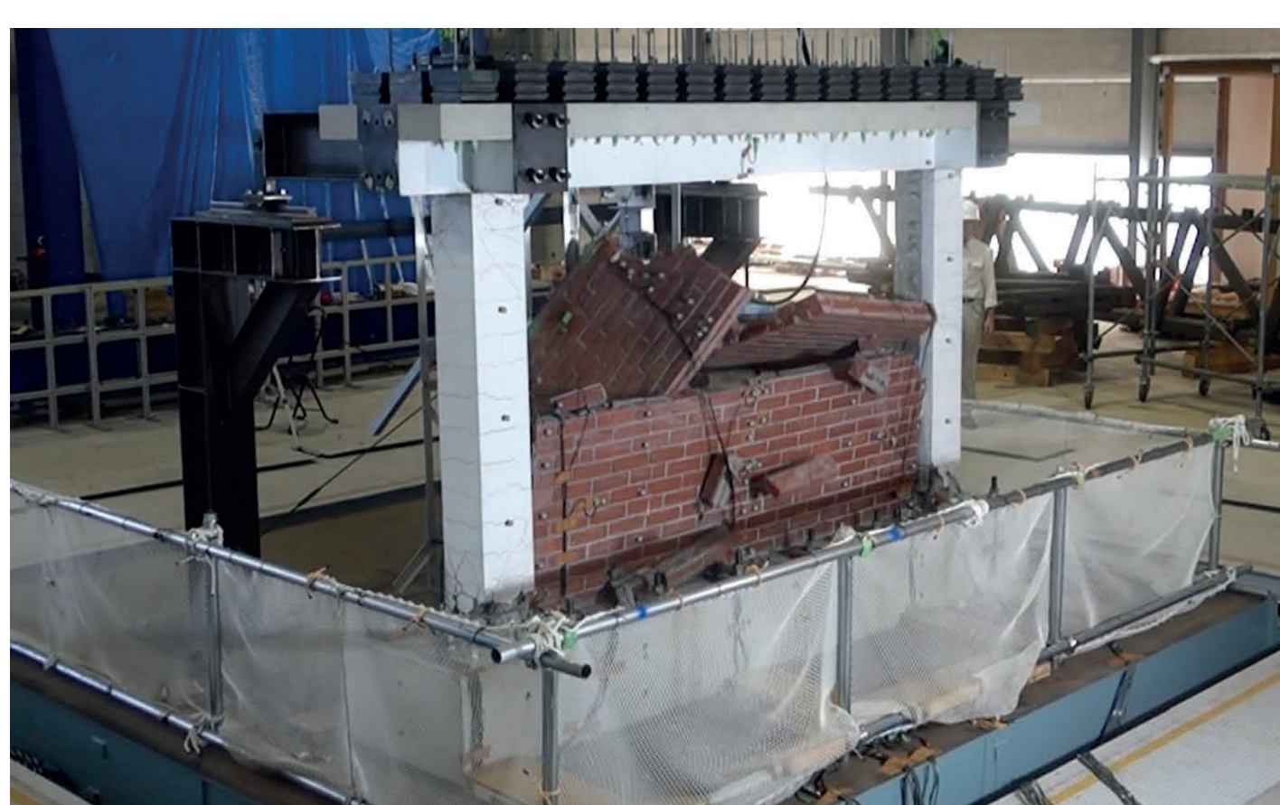
面外振動実験による組積造壁の崩壊
