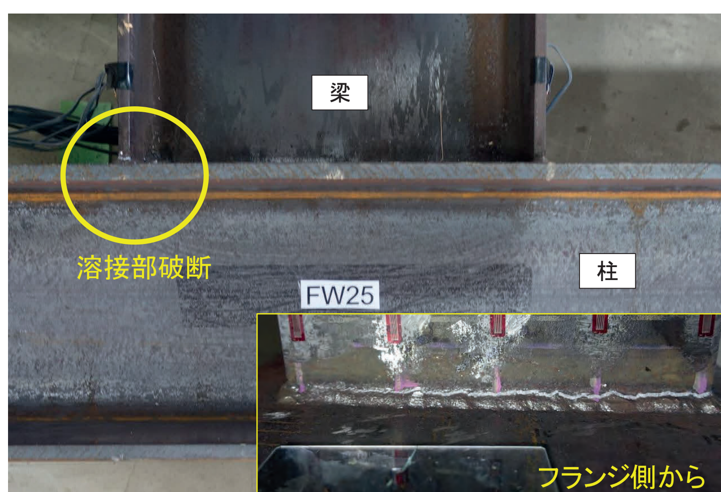
破壊実験による性能検証
