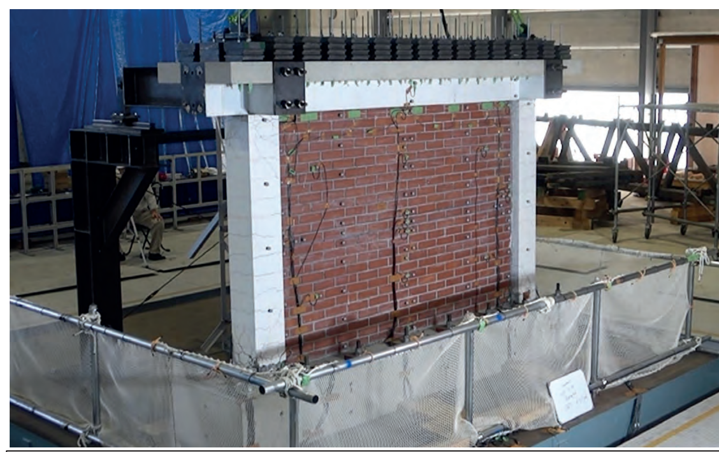
面内損傷を与えてから面外加振を行い、面内損傷が面外転倒へ与える影響を確認→途上国の地震被害低減への貢献
