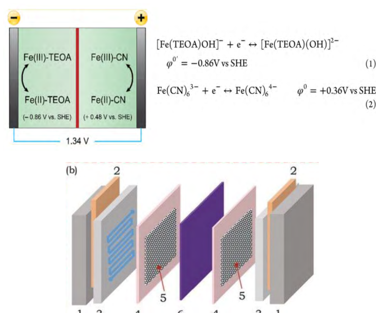
鉄レドックスフロー電池の高密度化
