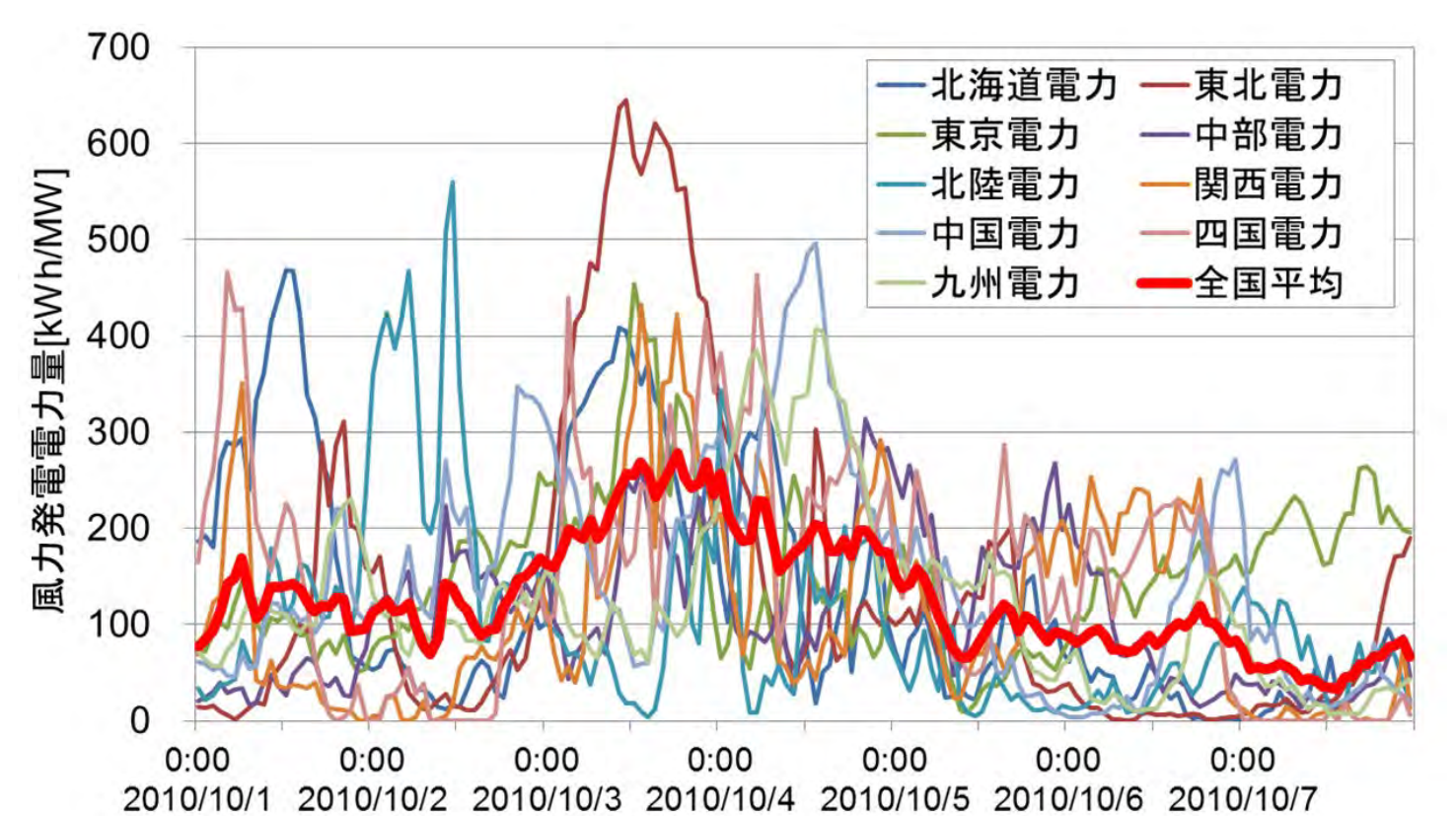
風力発電電力の変動例
