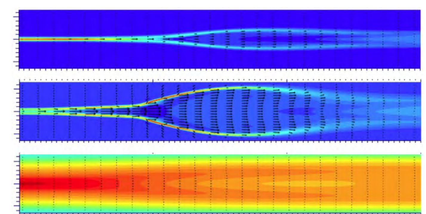
図3 磁気リコネクションによるジェット
