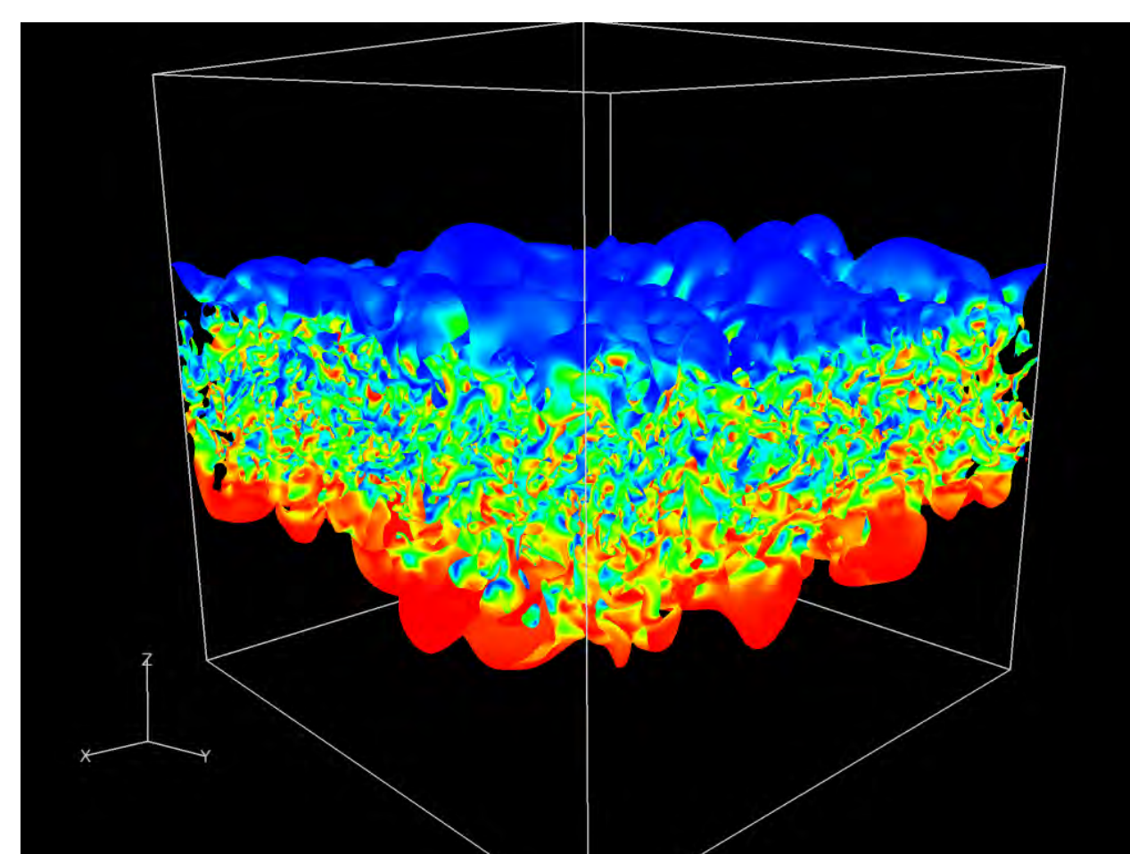
図2 回転系の乱流拡散の運動エネルギー
