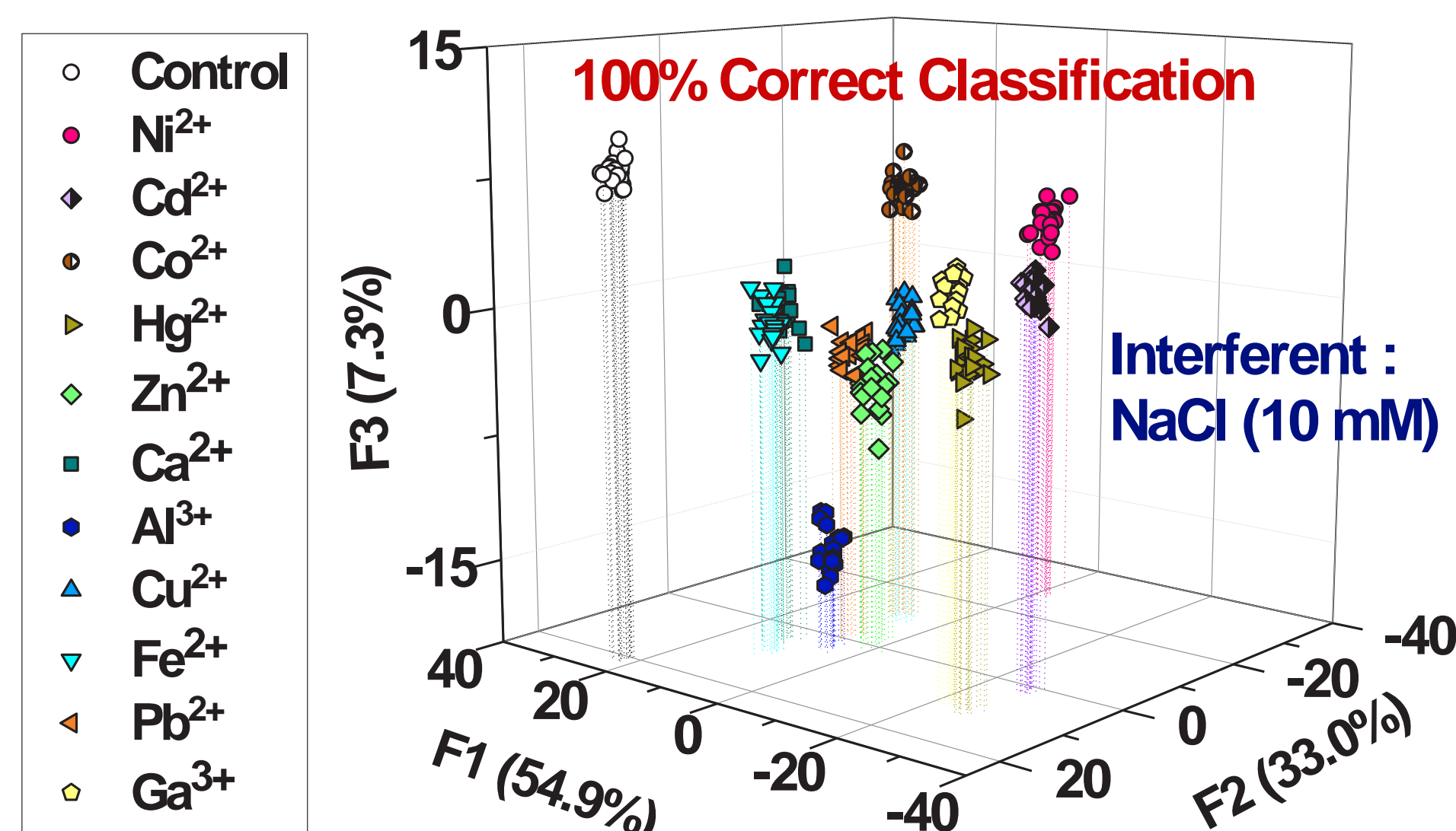
例：自己組織型比色ケモセンサアレイによる金属イオン類の同時定性分析
