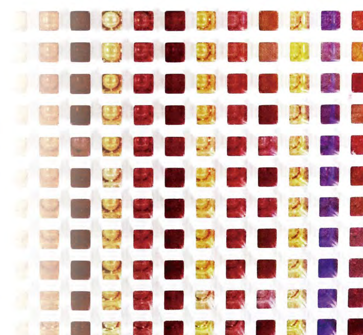
Chemosensor Array
