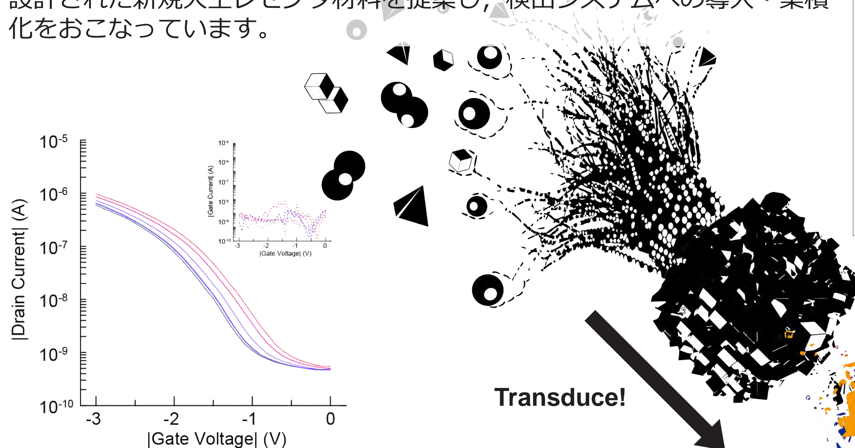
例：有機トランジスタ型化学センサによる単糖類の電氣的検出
