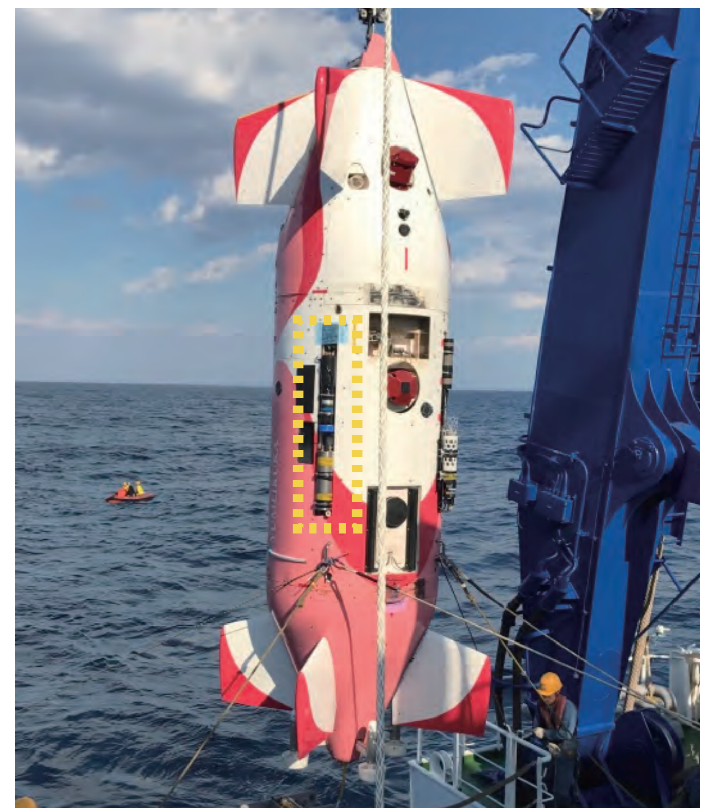
無人探査機に搭載された現場型 ATP定量分析装置 (YK17-05)
