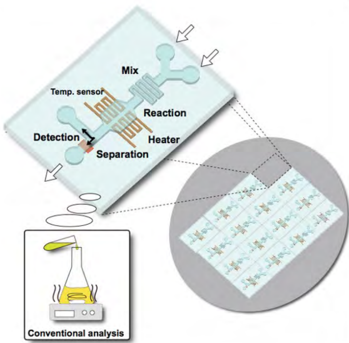
マイクロ流体システム概念図
