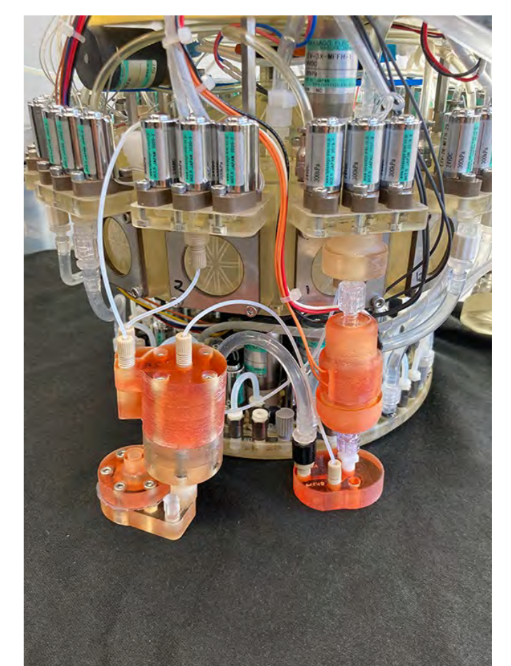
DNA抽出装置 (JAMSTEC)
