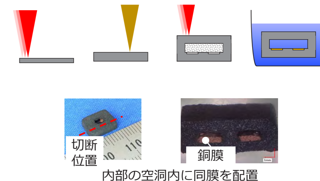
1. 造形 2. 活性化 3. 造形 4. メッキ
