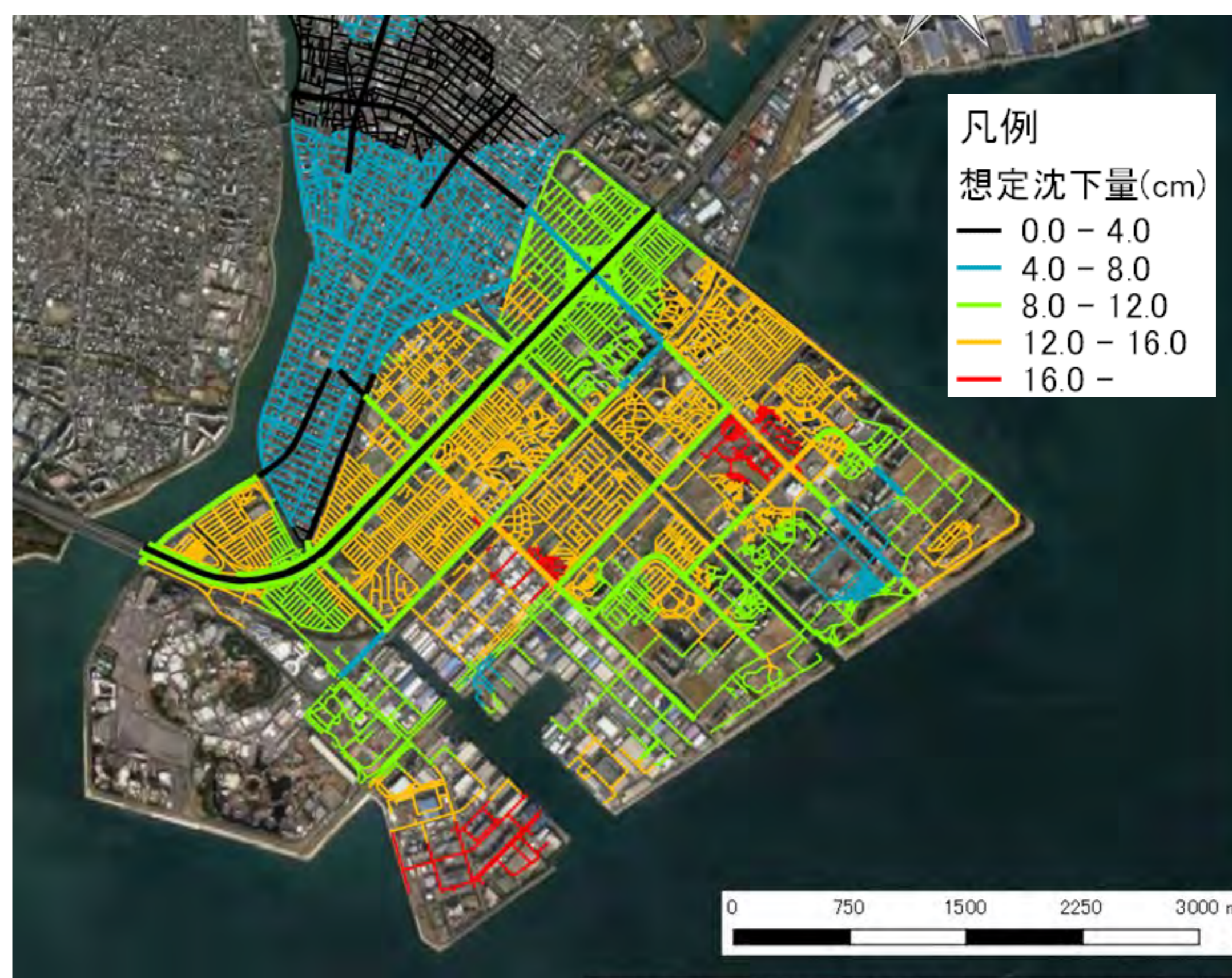
道路ネットワークの液状化ハザードマップの開発
