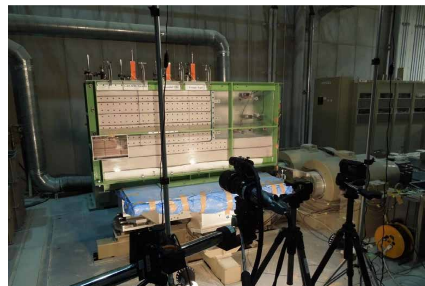
新素材を用いた補強土擁壁の耐震性に関する研究 補強効果を引抜き試験と振動台模型実験で検討
