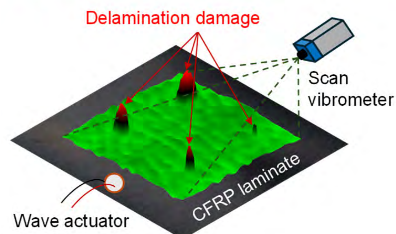
ガイド波の局所欠陥共振に基づくCFRP積層板中の剥離損傷の検出
