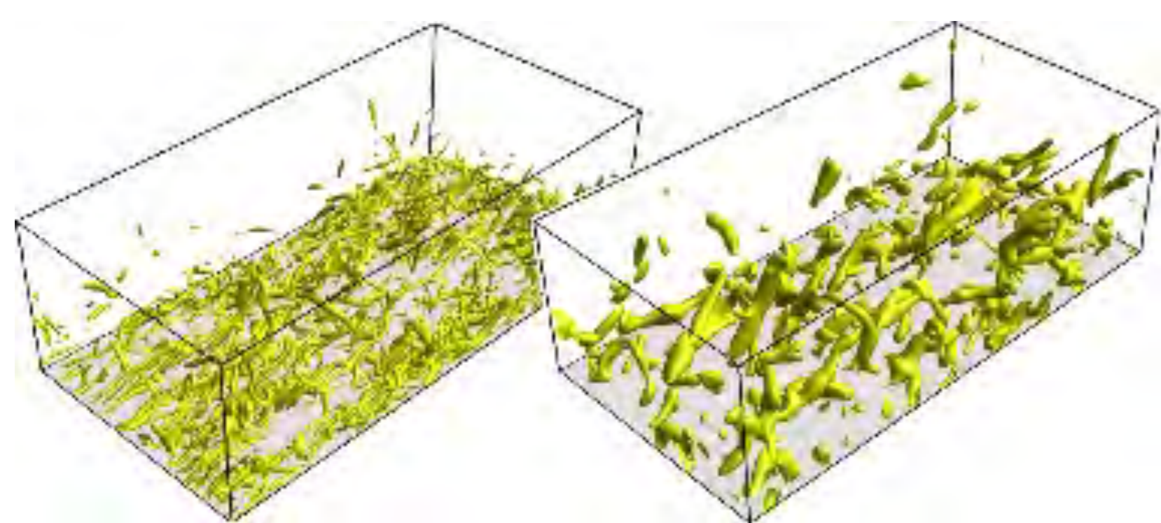
図1 チャンネル乱流の壁近くの渦構造
